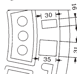
Spetthull tilpasset kombikrok/spettkrok og FV kroken
